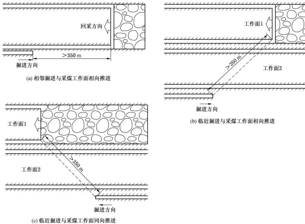
图 10 冲击地压危险煤层掘进与采煤工作面相隔距离要求
