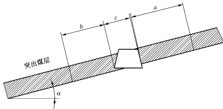
图 8 煤巷条带范围示意图
