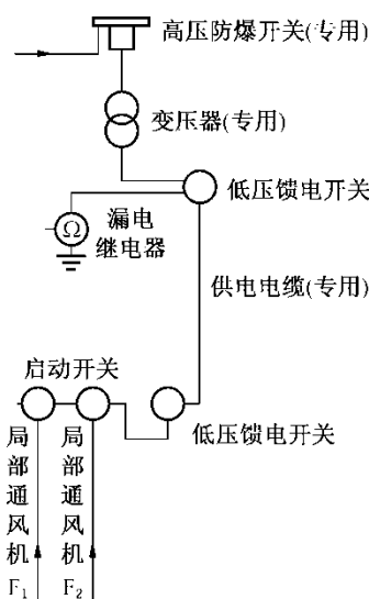
图6 “三专”简单供电系统图
