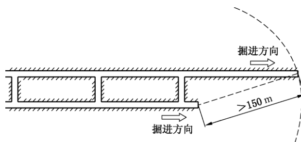
图 12 双巷掘进巷道错距示意图
