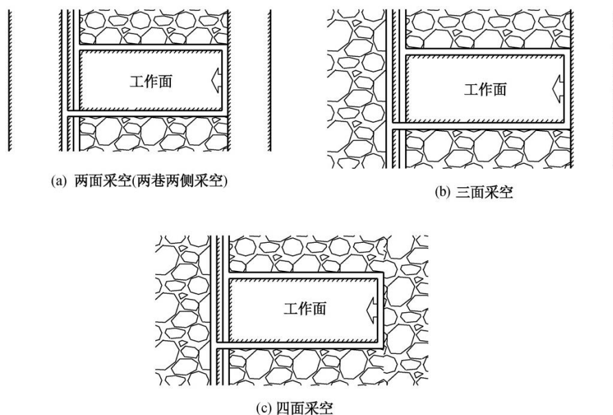
图 13 孤岛工作面（煤柱）布置示意图
