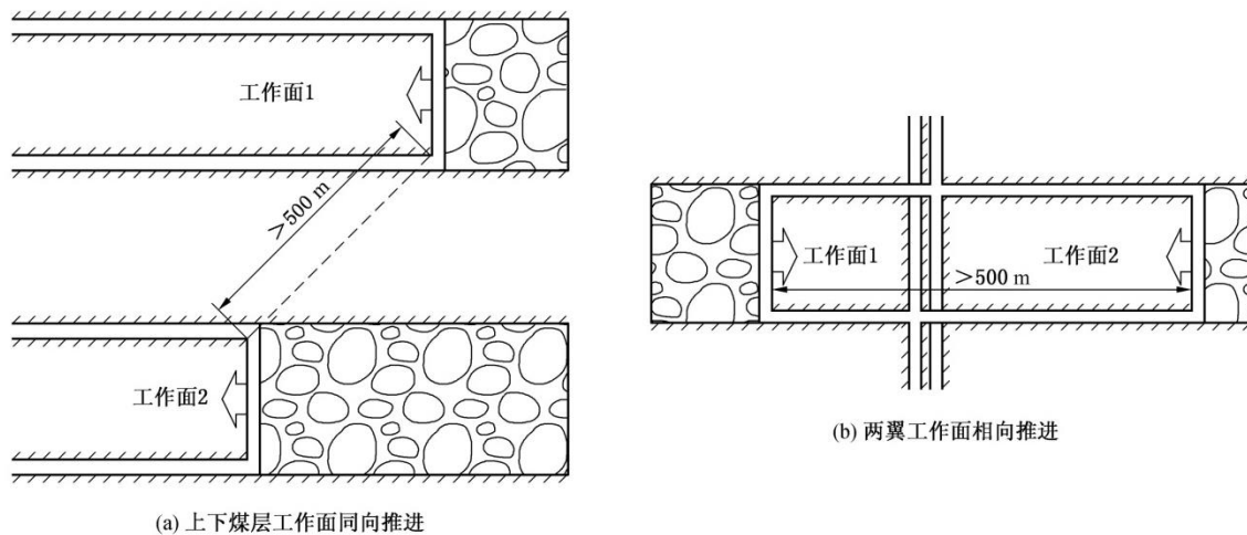
图 11 冲击地压危险煤层采煤工作面相隔距离要求
