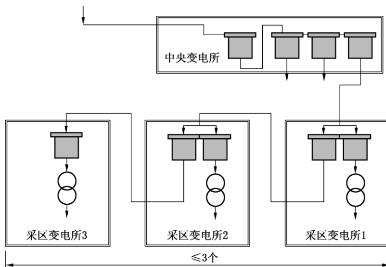
图 17 串接的采区变电所供电线路布置要求示意图
