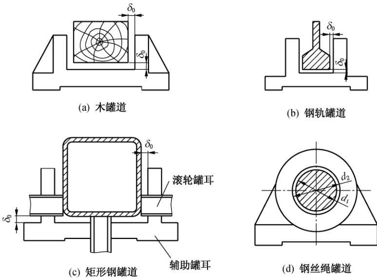
图 16 罐道和罐耳之间的间隙
