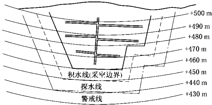
图 15 积水线、探水线、警戒线的划定
